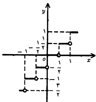
شکل ۷۶ : y = [2x]
