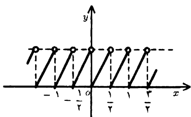
شکل ۷۸ : y = \{2x\}
