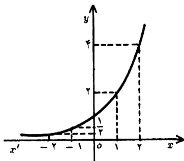
شکل ۳۶: نمودار تابع y = 2^x
