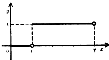
شکل ۸۱: y = [\sqrt{x}]
