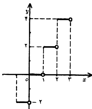
شکل ۷۷ : y = 2[x]
