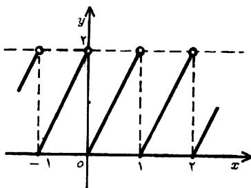
شکل ۷۹ : y = 2\{x\}
