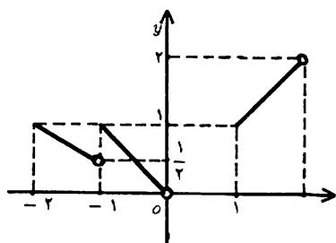
شکل ۸۰ : y = \frac{x}{[x]}
