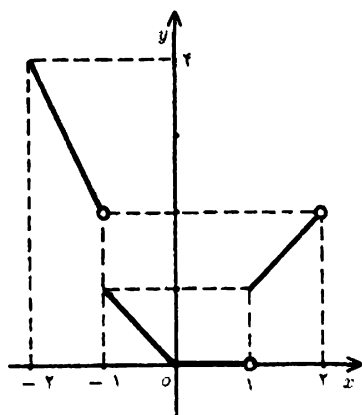
شکل ۸۲: y = x[x]
