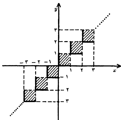
شکل ۸۳: [y] = [x]
